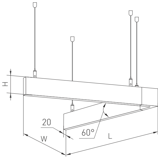
Рис. 1. Чертеж и габаритные размеры
