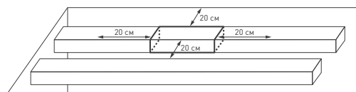
Рисунок 3. Свободное пространство вокруг источника
